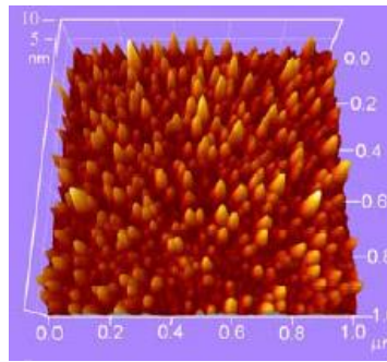
Image AFM 2D de nanoparticules obtenues par anodisation en régime intermédiaire électropolissage/prosification (Tetyana Nysyporuk, thèse LPM/INSA-Lyon, 2006)
