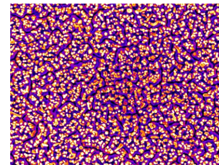
Cartographie AFM de nanofils d'oxyde au milieu d'une matrice de silice
